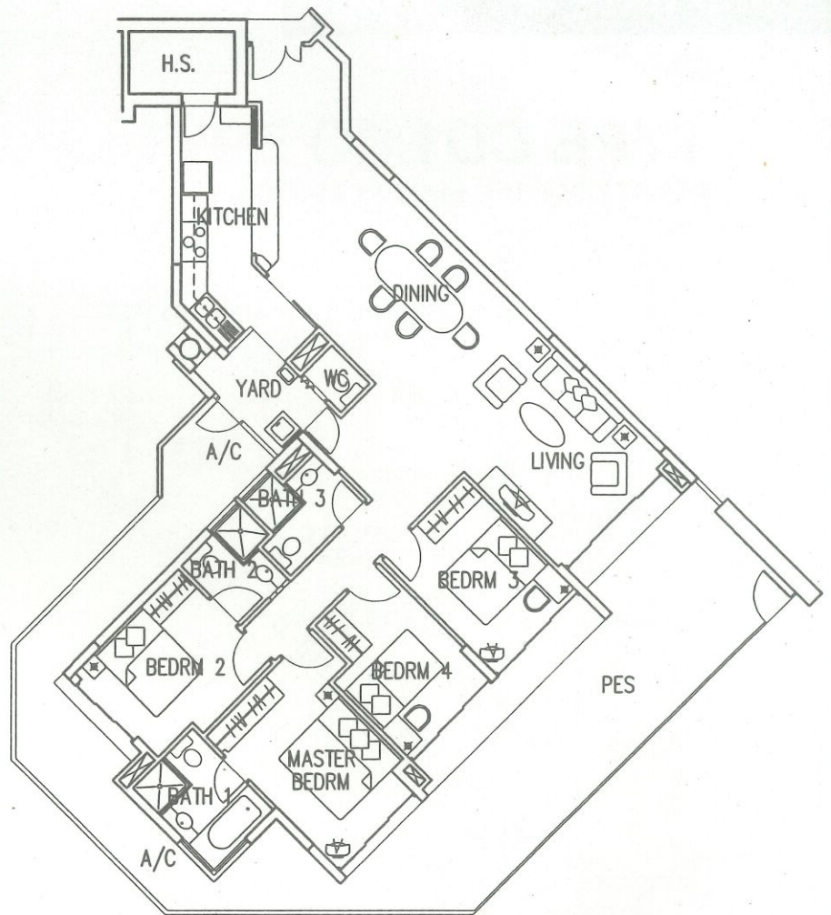
TYPE D1P1
